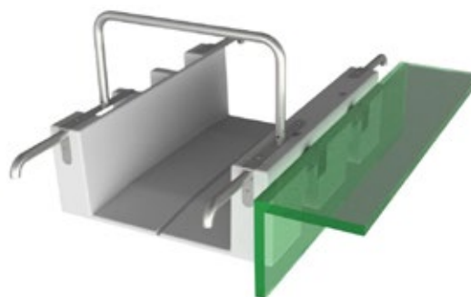
Rys. nr 7 Najazd/slip dla kajaków - zestawienie z zestawieniem ze stalowymi łącznikami uniwersalnymi do połączenia z nabrzeżem lub pomostem stałym
