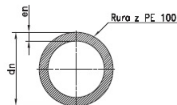
GAZ PE100
